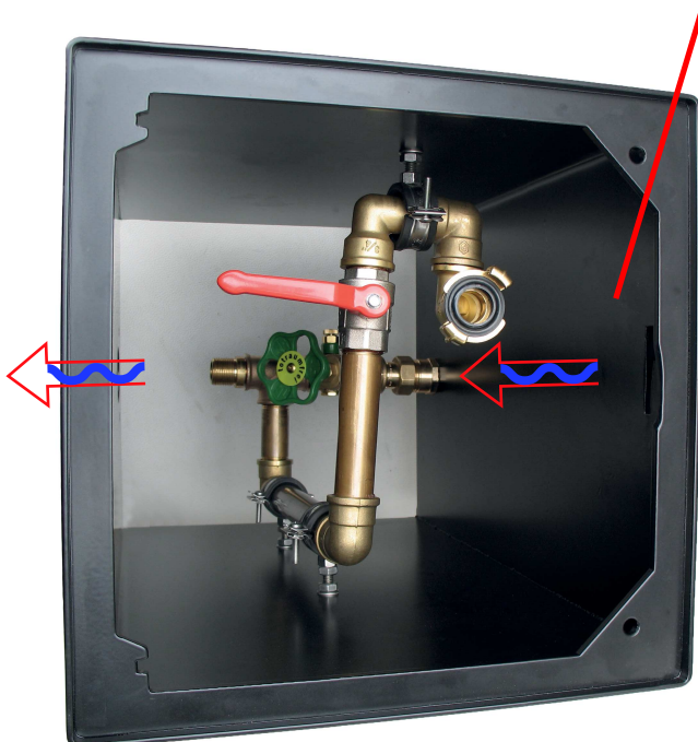
Zuleitung-Anschluss 1"
